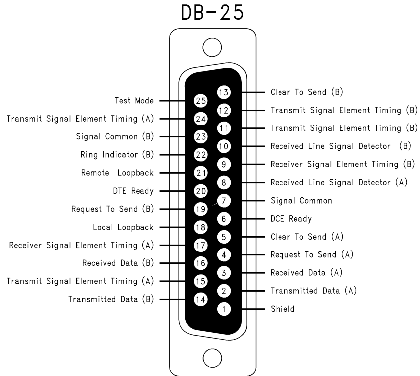
FIGURE 5. EIA/TIA-530-A DB-25
