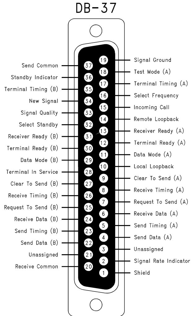
FIGURE 3. RS-449 DB-37
